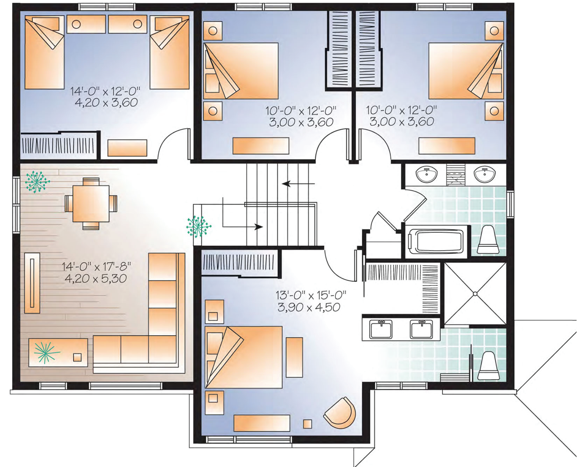
SECOND FLOOR PLAN DEUXIÈME PLANCHER
